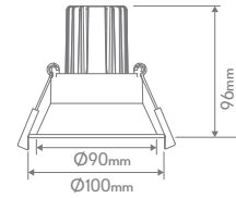
Cutout: \varnothing 90-92\text{mm} DT90 Tiltable to 15°
