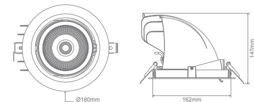
Cutout: Ø160mm - Ø170mm
