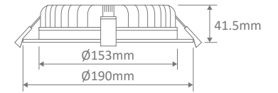
Cutout: Ø160 - Ø170mm
