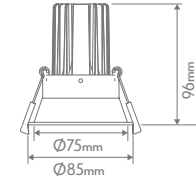
Cutout: \varnothing 75-77\text{mm}
