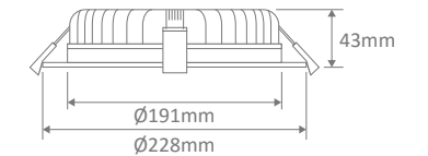
Cutout: Ø200 - Ø210mm
