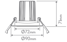
Cutout: \varnothing 72-75\text{mm} Tiltable to 15°
