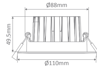
Tilt: 30° Cutout: Ø90-95mm
