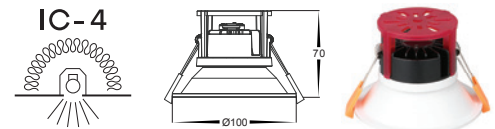
OPTIONAL IC4 CAP
