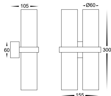
HV10592T
