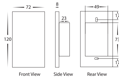
HV9220-3
