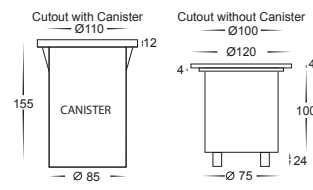
HV1801T HV1806T
