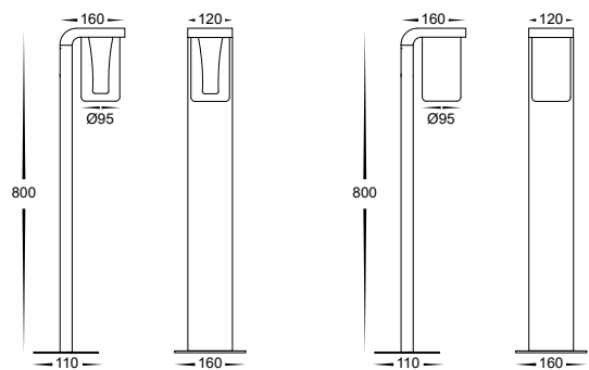
HV1692W-BLK Angela
