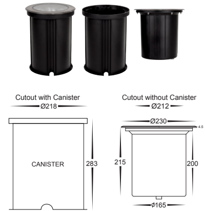
Face: 230mm Tilt: 15° HV1829T
